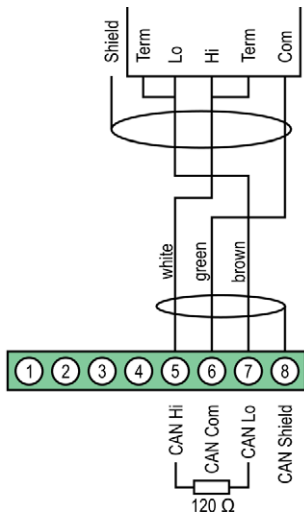
Stecker für CAN-Schnittstelle am PowerView3
