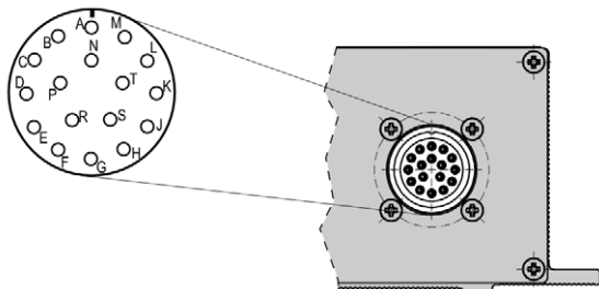
17-poliger Anschlussstecker (Ansicht von außen)
