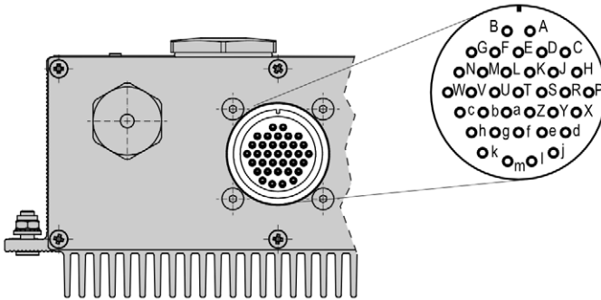
35-poliger Ausgangsstecker (Ansicht von außen)
