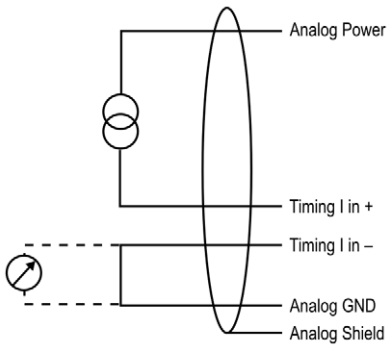
Zwei-Draht-Transmitter
