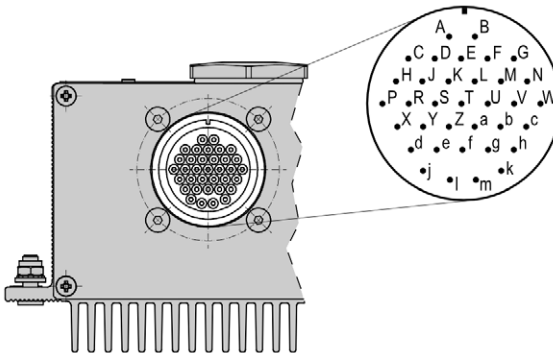
35-poliger Eingangsstecker (Ansicht von außen)
